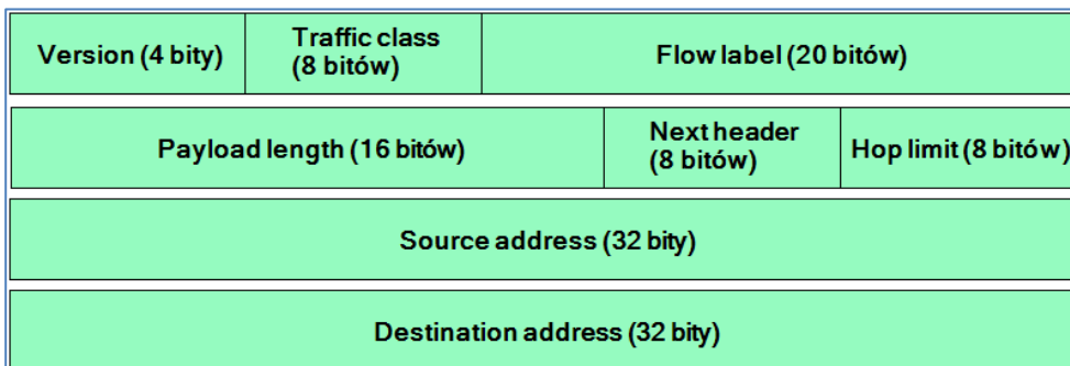
Rysunek 3.1 Nagłówek pakietu IPV6
