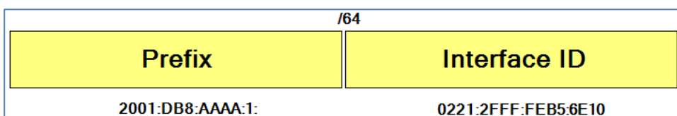
Rysunek 3.12 Przykładowe dynamiczne tworzenie prefiksu i ID interfejsu
